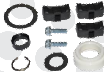
10827 da partida M-93 12V Prestolite Indiel/Mercedes/ Ford/VW
