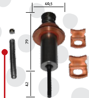
10717 do êmbolo da chave magnética da partida (parafuso M10) Nipodenso/Topic/Besta
