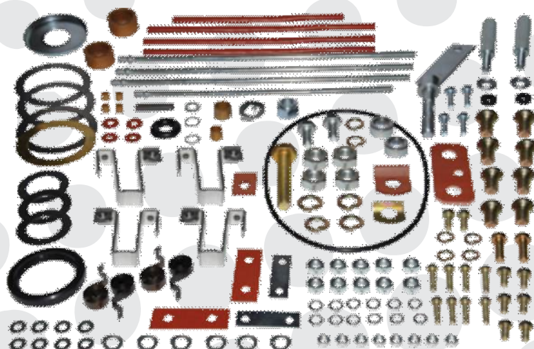
10880 kit completo de reparo da partida KB Bosch/Mercedes
