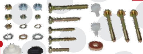
11672 do alternador para fixação das tampas, regulador e bornes de saída Delco/Chevette
