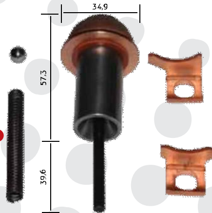
10812 do êmbolo da chave magnética da partida (parafuso M8) Nipodenso/Empilhadeiras/Toyota/Mitsubishi/Hitachi
