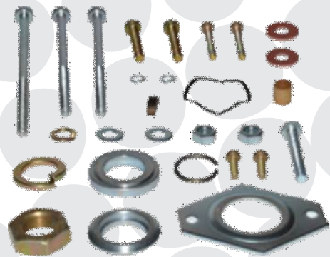
11769 kit do alternador Caterpillar c/ parafuso saída e fechamento Bosch/Caterpillar
