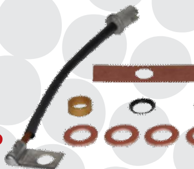
*10294 conexão da saída da bobina com o automático pino de latão, cabo e terminais de cobre Bosch/Ford/Chevrolet/VW
