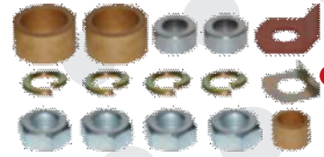
10623 calços dos bornes do mancal KB Bosch/Mercedes
