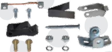
10652 porta escova com suporte, mola e cabo de ligação Delco/GM/Opala
