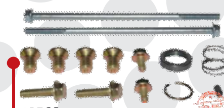
10568 reparo da partida 39MT GII - 24V Delco/Case/Fiat Allis/CNH Colheitadeira
