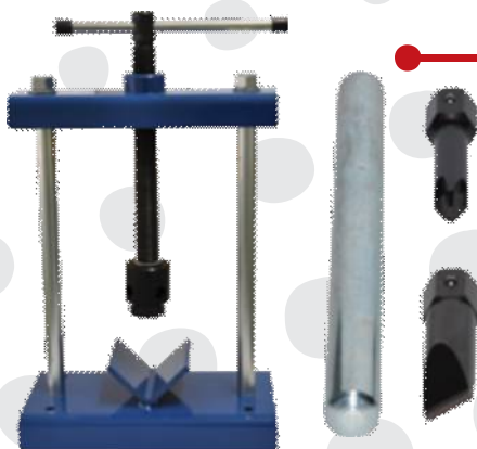
39503 saca rolamento 6003 com defletor plástico Alternador Bosch 80 amp. eletrônico (necessário GB 39895)
