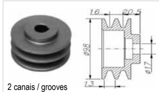
2 canais / grooves
