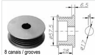
8 canais / grooves
