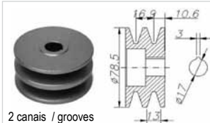
2 canais / grooves
