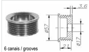
6 canais / grooves
