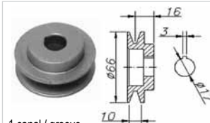
1 canal / groove
