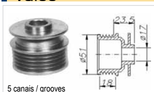
5 canais / grooves
