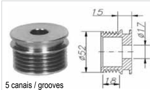
5 canais / grooves
