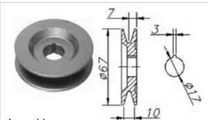
1 canal / groove
