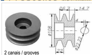
2 canais / grooves
