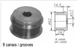
8 canais / grooves
