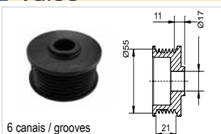
6 canais / grooves
