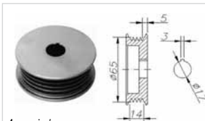
4 canais / grooves
