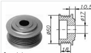
5 canais / grooves
